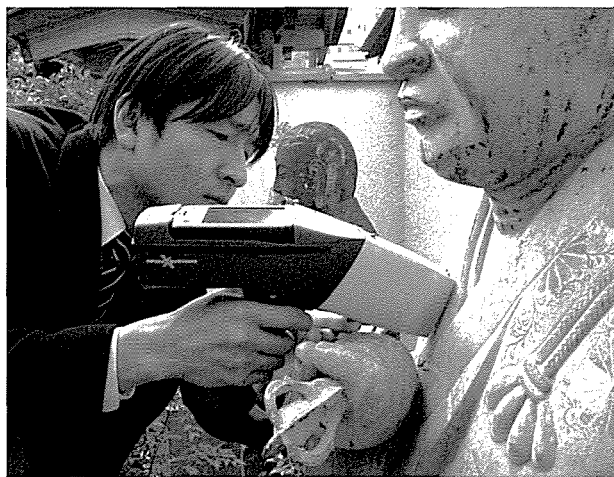
写真M-4 可搬型分析装置による作業状況
